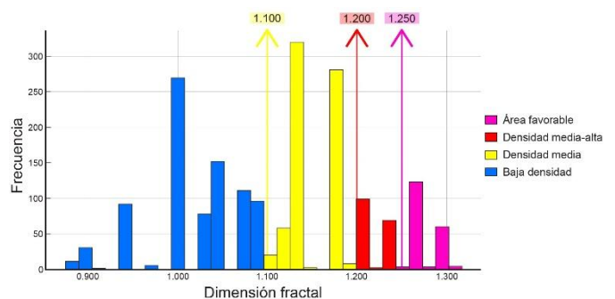
Figura 5. Clasificación Fractal de Densidad Estructural: Identificación de Áreas Potencialmente Favorables
