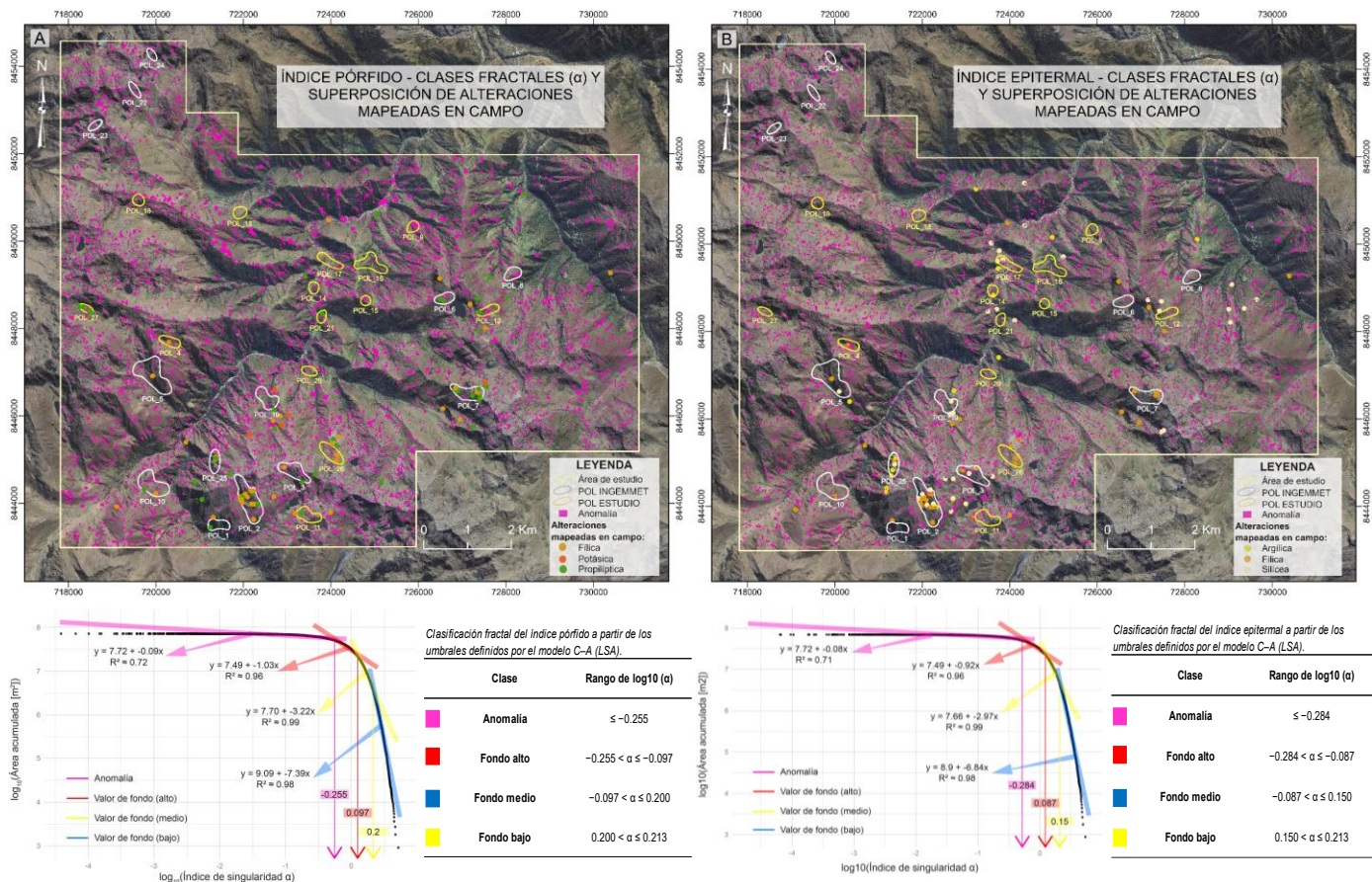
Figura 10 Mapas fractales de índices espectrales y su validación con alteraciones mapeadas en campo. a) Índice Pórfido: clases fractales ( \alpha ) y superposición de alteraciones hidrotermales (filica, potásica, propilítica); b) Índice Epitermal: clases fractales ( \alpha ) y superposición de alteraciones (argílica, filica, sílica). Debajo se muestran las curvas C–A y los umbrales fractales definidos para cada índice.
