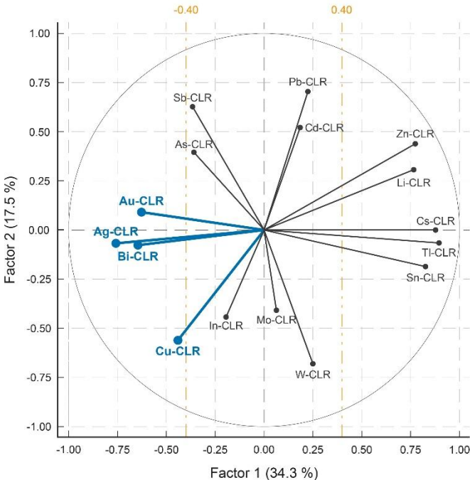
Figura 2. Biplot F1–F2 (rotación Varimax) a partir de datos transformados mediante CLR, que muestra la agrupación de elementos guía de mineralización (Cu, Au, Ag, Bi).
