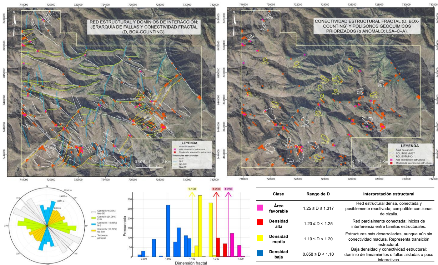
Figura 9 Análisis estructural fractal y conectividad de fallas. a) Red estructural y dominios de interacción jerarquizados mediante box-counting; b) conectividad estructural fractal (D) integrada con polígonos geoquímicos priorizados ( \alpha anómalo, LSA–C–A).
